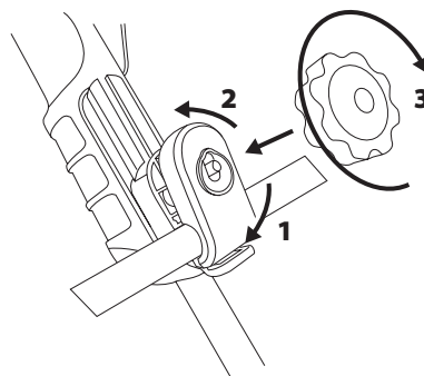
Réglage de la hauteur et de la position du guidon
